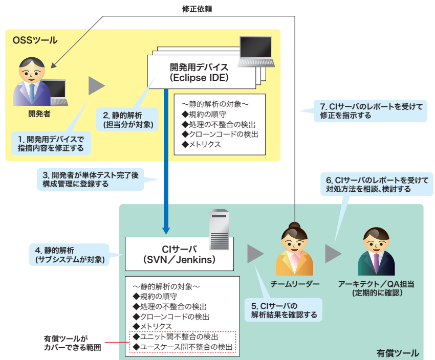
図 SOMPOシステムイノベーションズが検討した静的解析ツールの活用方法 (出典:SOMPOシステムイノベーションズ資料)
